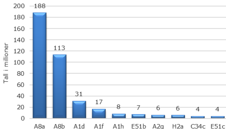
Figur 7: Topp ti takster, Manuellterapeuter
